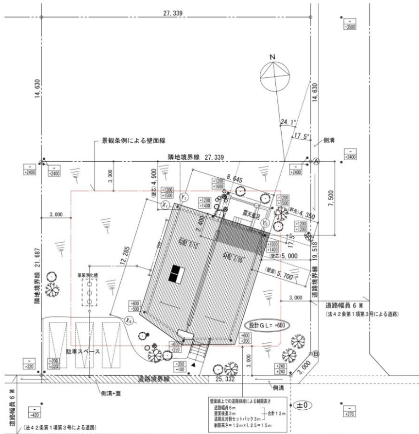
配置図
